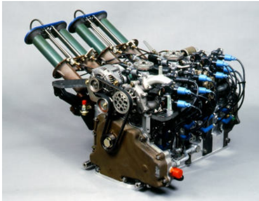
R26B 4-rotatiemotor in de Mazda 787B
